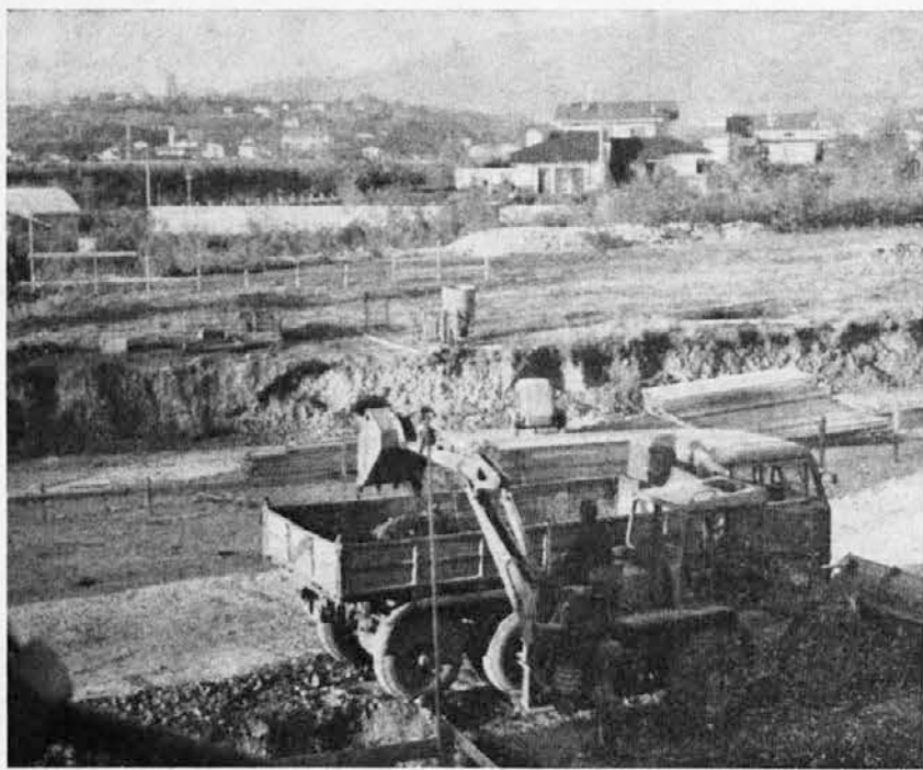
Predeno so zrastle temelji novega Zavoda sv. Družine, je bilo treba pripraviti teren z izkopom prodnatega pa tudi skalnatega zemljišča
